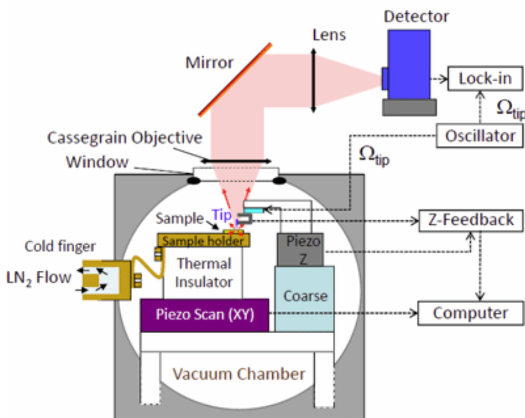
Image d'un sNSOM à basse température (Appl. Phys. Lett. 98, 231112 (2011)).
